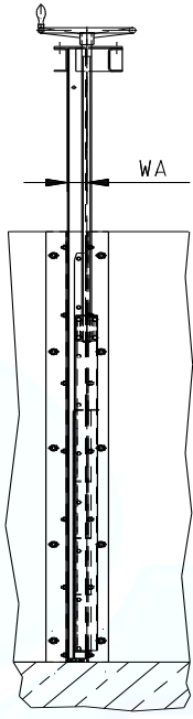
Schnitt B-B
