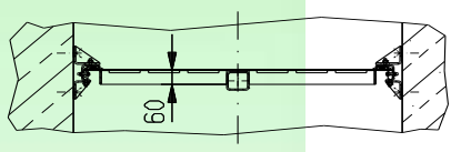
Schnitt A-A
